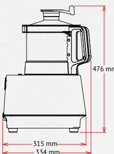
Vista laterale
