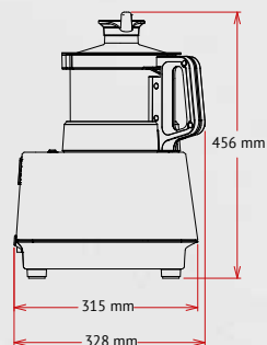
Vista laterale
