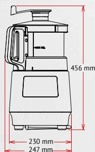
Vista frontale
